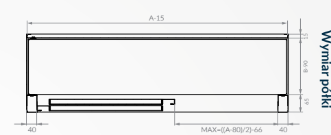
PRZEKRÓJ-WIDOK Z GÓRY Wymiar półki
