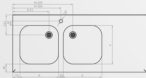
RZUT Z GÓRY
