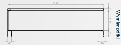
PRZEKRÓJ-WIDOK Z GÓRY Wymiar półki
