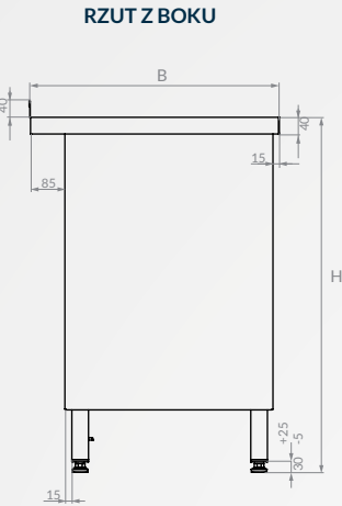
RZUT Z BOKU
