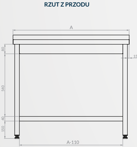
RZUT Z PRZODU
