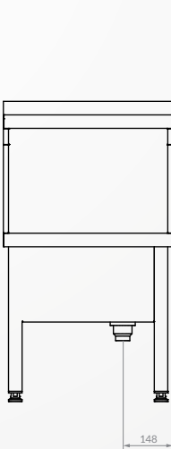
RZUT Z PRZODU
