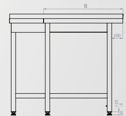
RZUT Z BOKU
