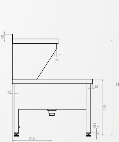
RZUT Z BOKU
