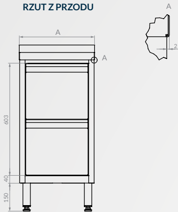
RZUT Z PRZODU
