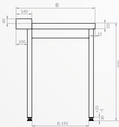
RZUT Z BOKU
