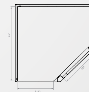
PRZEKRÓJ-WIDOK Z GÓRY
