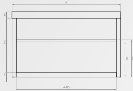
RZUT Z PRZODU
