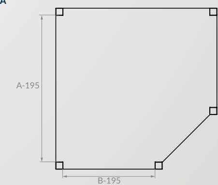
RZUT Z GÓRY PÓŁKA
