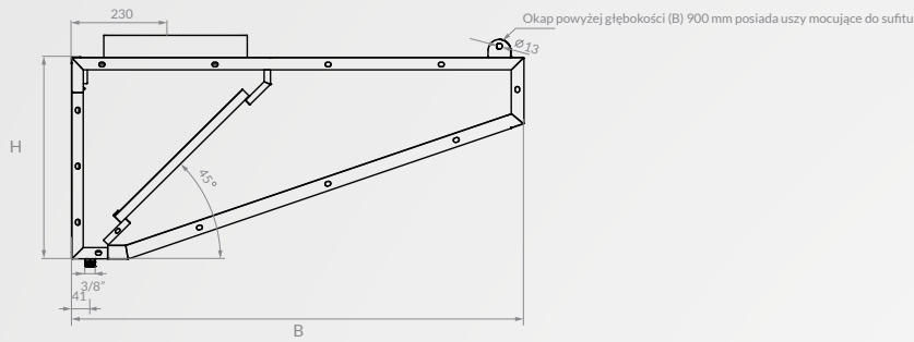
RZUT Z BOKU
