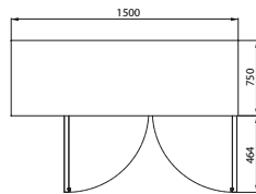
TTP6-180-20 GLASS
