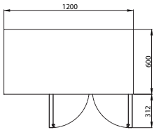
TTP6-120-20 TTN6-120-20
