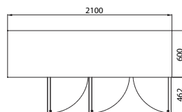
TTP6-210-30 TTN6-210-30
