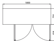
TTP7-120-20 GLASS
