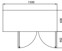
TTP6-150-20 TTN6-150-20
